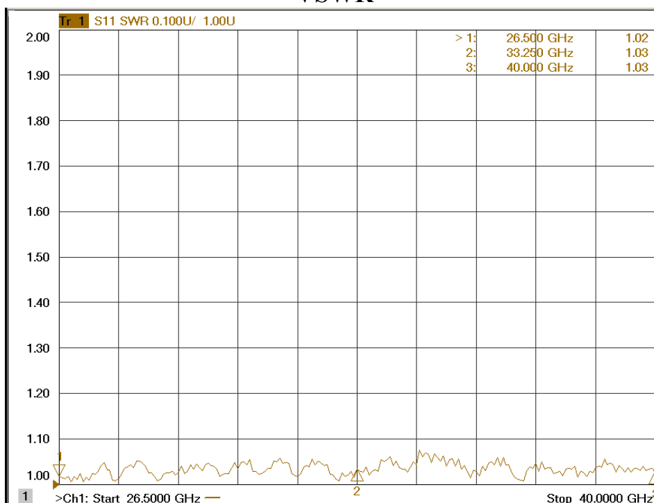
VSWR
