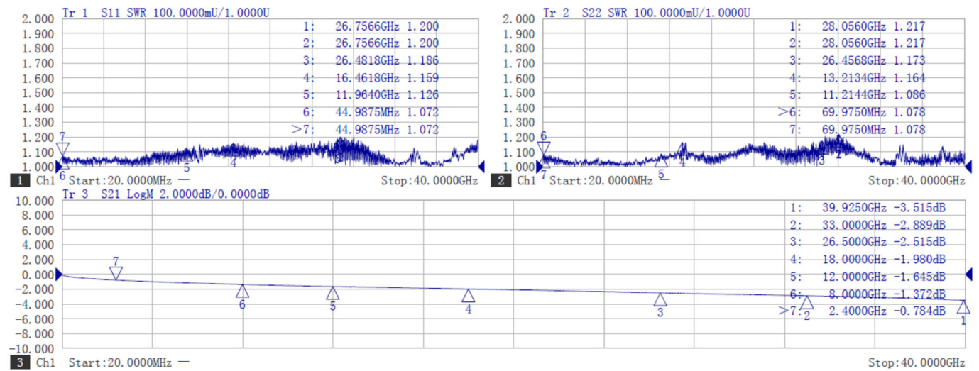
2.92mm(M)-2.92mm(F) 0.8M
