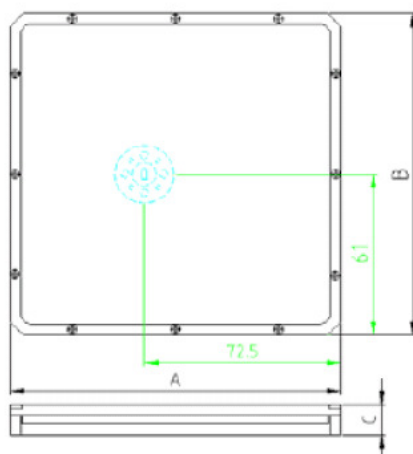
S-X : RLSA Antenna
