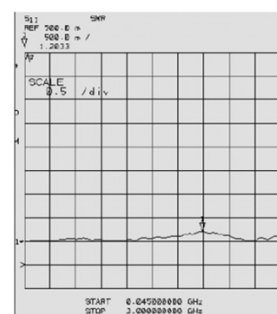
VSWR
