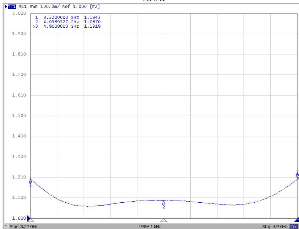
VSWR
