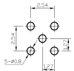
REFERENCE P.C.B LAYOUT
